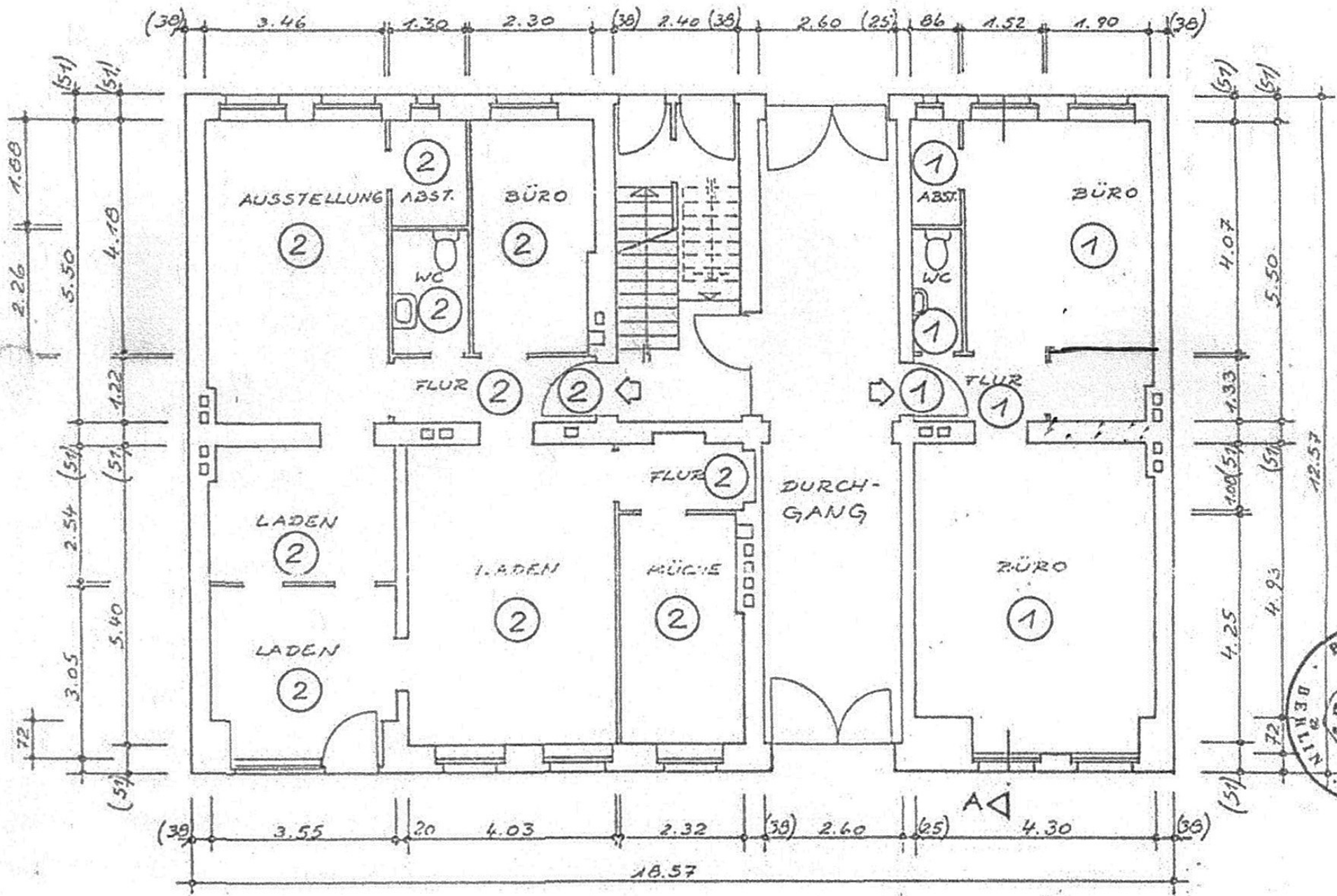
ERDGESCHOSS VORDERHAUS
